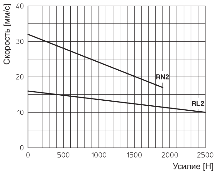
2-аходная трапецеидальная пара Тг 14 8 (P4)
