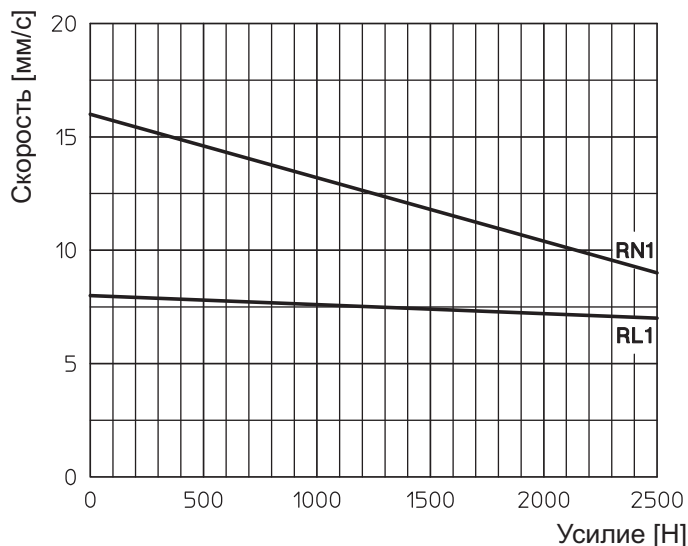
1-заходная трапецеидальная пара Тг 14 4
