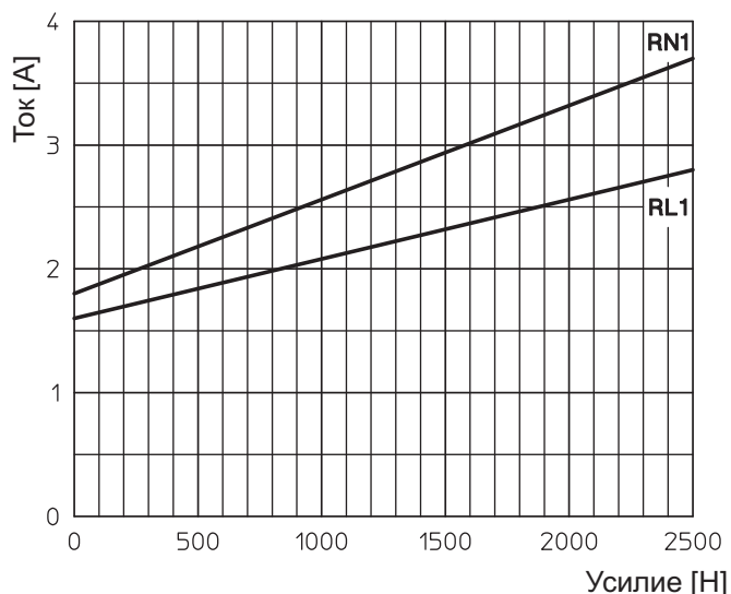
1-заходная трапецеидальная пара Тг 14 4
